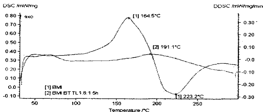
Hình 4. Giản đồ DSC của BMI (đường 1) và BMI.BT. 1,6:1. 5h (đường 2)
