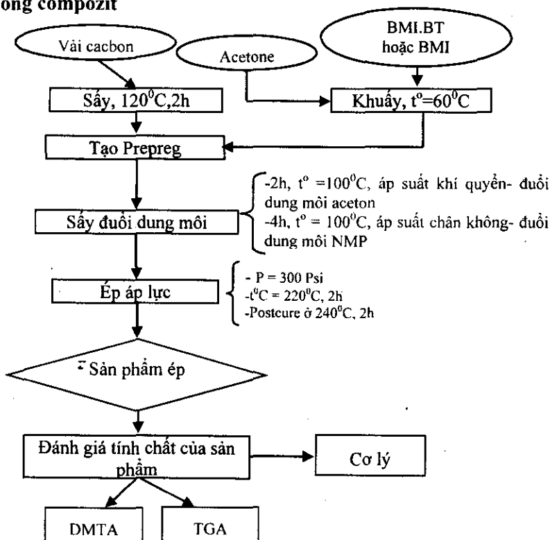
Hình 3. Sơ đồ quá trình gia công compozit
