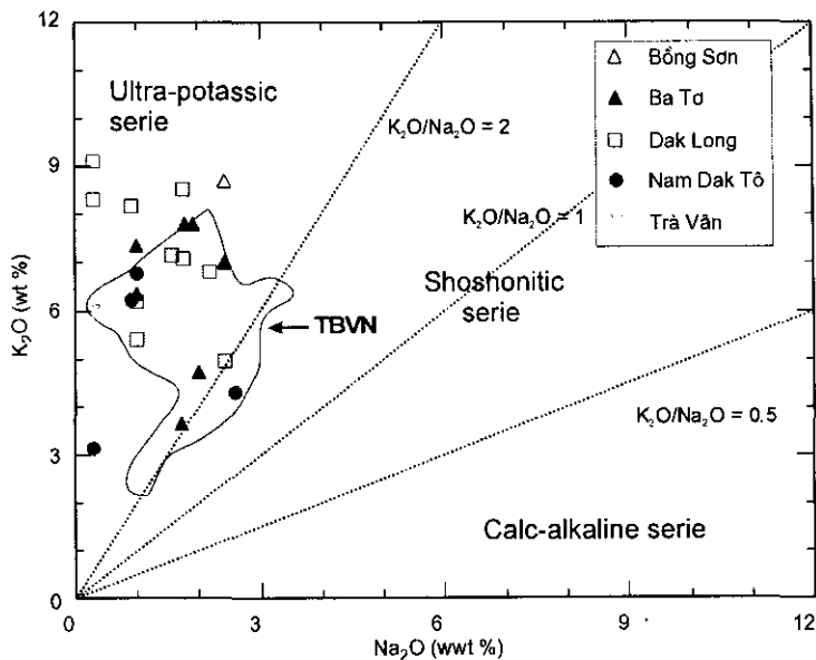
Hình 2. Tương quan \text{Na}_2\text{O}+\text{K}_2\text{O} của các đá lamprophyr MT&TN, so sánh với các đá lamproit TBVN [1]
