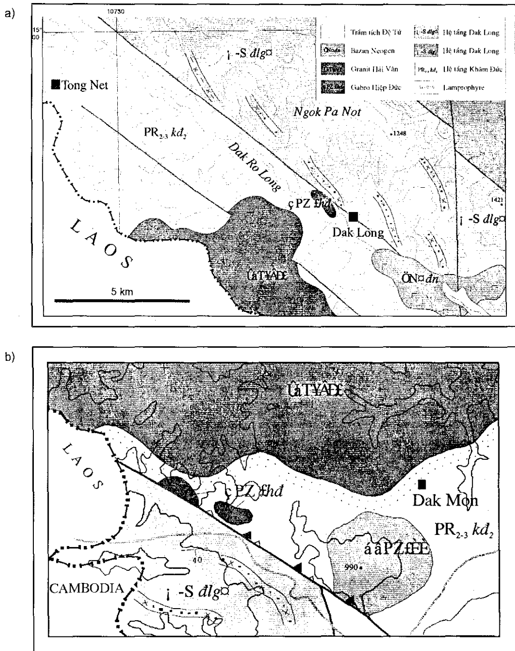
Hình 1. Sơ đồ phân bố một số thành tạo lamprophyr MTVN a) Dak Long, b) Dak Mon (trên cơ sở bản đồ Địa chất tỷ lệ 1:200.000)
