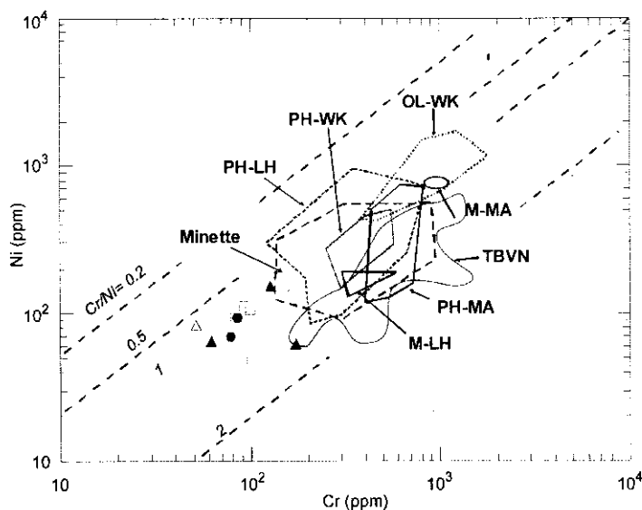
Hình 4. Tương quan Ni - Cr của các đá lamprophy MT&TN (các trường theo [9]). Ký hiệu như hình 3.
