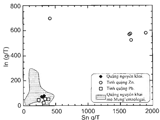
Hình 2. Biểu đồ tương quan hàm lượng In-Sn trong quặng nguyên khai, tinh quặng kẽm và tinh quặng chì các mỏ chì-kẽm khu vực Chợ Đồn
