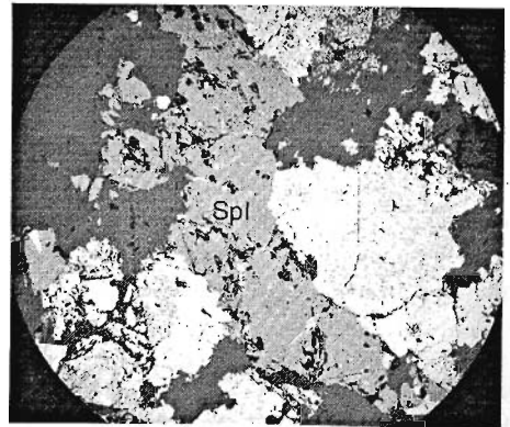
Ảnh 3. Khoáng vật sphalerit (Spl) có kiến trúc phân rã dung dịch cứng (mẫu NB08-08)
