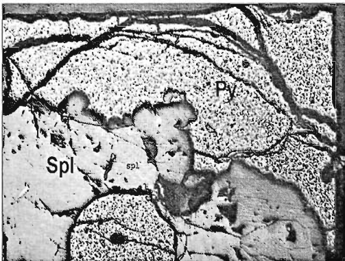
Ảnh 4. Khoáng vật pyrit (Py) với mặt sản đặc trưng và bị gặm mòn bởi sphalerit - Spl (mẫu KC 1053)
