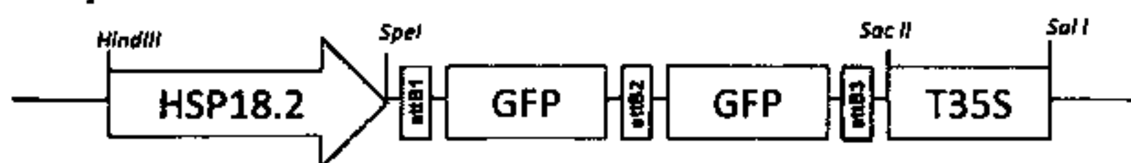
Hình 4. Sơ đồ cấu trúc vector pXK7FNF2.0/HSP18.2
