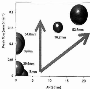
Biểu đồ 04. Xu hướng quan hệ giữa đỉnh lũ và chỉ số mưa trước đó 2 ngày (API2)
