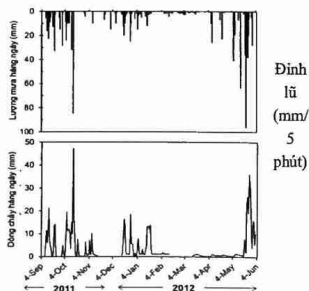
Biểu đồ 03. Phân ứng của dòng chảy lưu vực với lượng mưa
