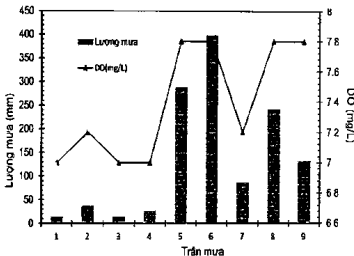
Biểu đồ 11. Đặc điểm lượng oxy hòa tan của dòng chảy lưu vực và lượng mưa
