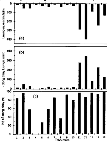
Biểu đồ 05. Đặc điểm mưa (a), dòng chảy lưu vực (b) và hệ số dòng chảy lưu vực (c) theo trận mưa
