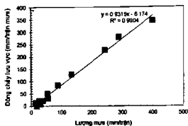
Biểu đồ 06. Quan hệ giữa lượng mưa và dòng chảy lưu vực
