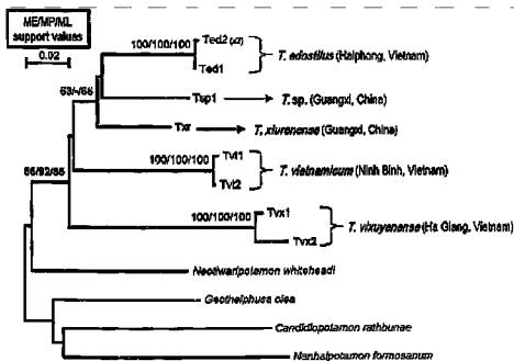
Hình 1: Cây tiến hóa cho giống Tiwaripotamon ở Việt Nam và Trung Quốc (cùng một số loài thuộc giống khác có quan hệ gần gũi với giống Tiwaripotamon ) (Nguồn: Shih et Do, 2014)
