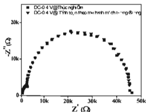
Hình 7. Phổ tổng trở Nyquist thực nghiệm và tính toán theo mô hình mạch tương đương của chuyển tiếp SnO 2 /CNTs ở chế độ phân cực ngược DC - 0,4 V.
