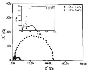
Hình 4. Phổ tổng trở Nyquist của chuyển tiếp SnO 2 /CNTs ở điện áp phân cực DC ± 0,4 V tại nhiệt độ phòng.
