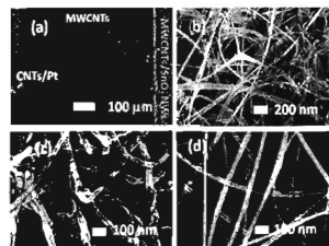
Hình 2. Ảnh FE-SEM của chuyển tiếp SnO 2 /CNTs trên điện cực Pt (a), ảnh phóng đại của chuyển tiếp (b), ảnh phóng đại cao của CNTs (c), ảnh phóng đại cao của SnO 2 trên điện cực Pt (d).
