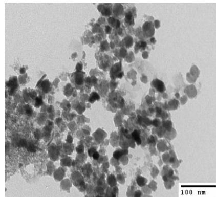
Hình 3. Nghiên cứu XRD và TEM của mẫu \text{NiFe}_2\text{O}_4 sau khi thủy nhiệt tại 120^\circ\text{C}
