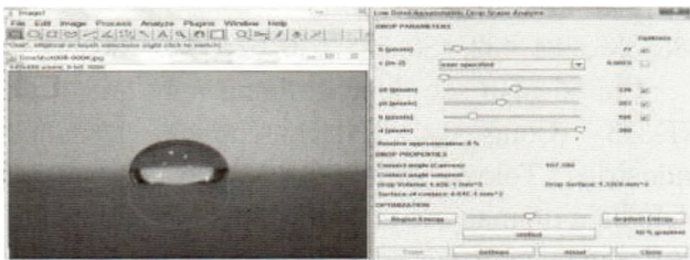
Hình 2. Đo góc tiếp xúc của giọt nước bằng phần mềm ImageJ
