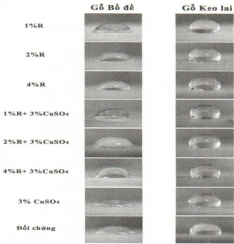
Hình 3. Hình ảnh góc tiếp xúc của giọt nước trên bề mặt gỗ được xử lý bởi hỗn hợp keo nhựa thông - đồng sunphat
