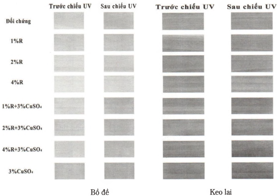
Hình 6. Hình ảnh bề mặt gỗ được xử lý bởi hỗn hợp keo nhựa thông - đồng sunphat trước và sau chiếu UV Trước khi chiếu UV, các giá trị L^* , a^* , và b^* của mẫu gỗ Bồ đề không xử lý (đối chứng) tương ứng là 81,60, 7,70 và 22,83. Giá trị L^* của các mẫu gỗ đã ngâm tẩm dao động trong khoảng từ 74,73 – 79,33, giá trị a^* dao động từ 1,89 – 8,16 và giá trị b^* dao động từ 18,17 – 22,94. Kết quả cho thấy, gỗ Bồ đề sau khi được xử lý bởi dung dịch keo nhựa thông đơn lẻ, gỗ trở nên đỏ hơn và vàng hơn, tuy nhiên sau khi kết hợp keo nhựa thông - đồng sunphat để xử lý thì bề mặt gỗ trở nên xanh hơn và hơi sẫm hơn so với mẫu đối chứng và mẫu chỉ xử lý bởi keo nhựa thông đơn lẻ (Hình 6). Điều này là do sự có mặt của đồng trong dung dịch ngâm tẩm. Tuy nhiên, không giống với gỗ Bồ đề, sau khi được xử lý bởi dung dịch keo nhựa thông đơn lẻ hay kết hợp với đồng sunphat, màu sắc của bề mặt gỗ Keo lai không thay đổi nhiều so với mẫu không được xử lý (Hình 7). Các giá trị L^* , a^* và b^* của bề mặt mẫu gỗ Keo lai không xử lý tương ứng là 61,99; 9,68 và 19,73. Đối với mẫu gỗ đã ngâm tẩm có giá trị L^* dao động trong khoảng từ 56,18 – 65,06, giá trị a^* dao động từ 7,81 – 9,65 và giá trị b^* dao động từ 19,20 – 20,14. Sau khi chịu tác động của tia UV, màu sắc của bề mặt gỗ đã bị biến đổi nhiều trong khoảng 480 giờ đầu đối với gỗ Bồ đề (Hình 4) và trong 576 giờ đối với gỗ Keo lai (Hình 5), tuy nhiên khi thời gian chiếu tiếp tục tăng thì màu sắc của gỗ biến đổi rất ít hoặc gần như không biến đổi ở cả 2 loại gỗ thử nghiệm. Sau 720 giờ chiếu UV, các giá trị \Delta a^* và \Delta b^* đều có giá trị dương trong tất cả các mẫu không xử lý và các
