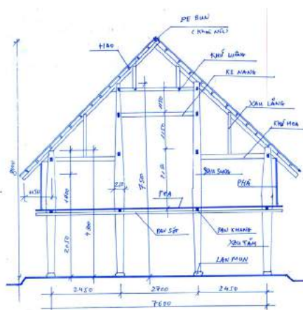
Vì kèo với liên kết kèo - xà - cột
