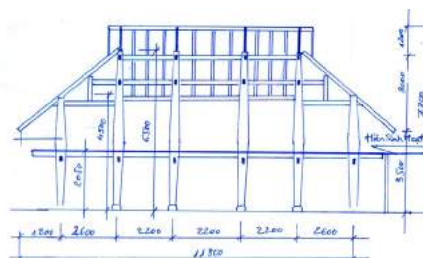
Vì kèo với liên kết kèo - xà - cột
