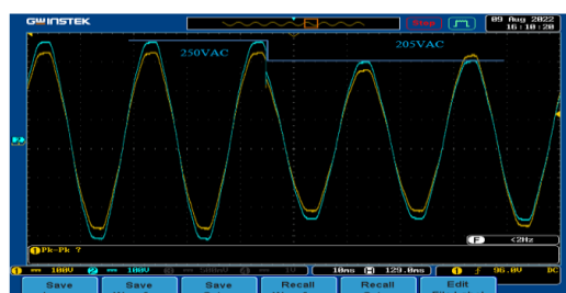
Hình 26. Điện áp tải khi nguồn cao - thấp
