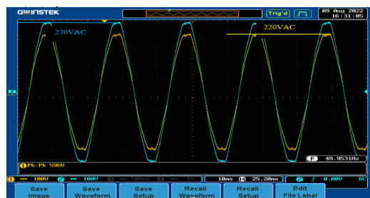
Hình 30. Điện áp tải với tải phi tuyến ở điện áp nguồn cao 270V
