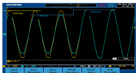
Hình 28. Điện áp tải khi nguồn thấp - ổn định
