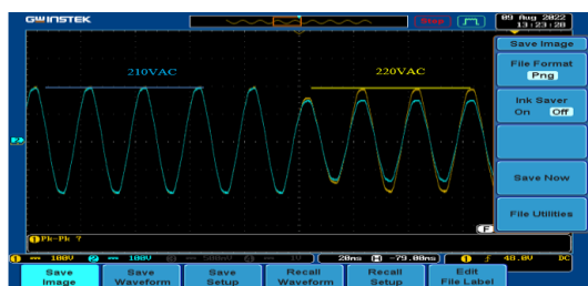
Hình 27. Điện áp tải khi nguồn ổn định – thấp
