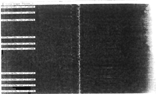
Hình 8. Đoạn băng ghi sonar tuyến T16A-3 thể hiện thành phần trầm tích đáy biển là bùn lẫn cát - vùng biển Phú Quốc - Hà Tiên, 2008.
