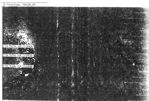
Hình 5: Đoạn băng ghi sonar tuyến T08-29A 05 thể hiện thành phần trầm tích đáy biển gồm cát, sạn sỏi - vùng biển ven bờ Sóc Trăng, 2008.
