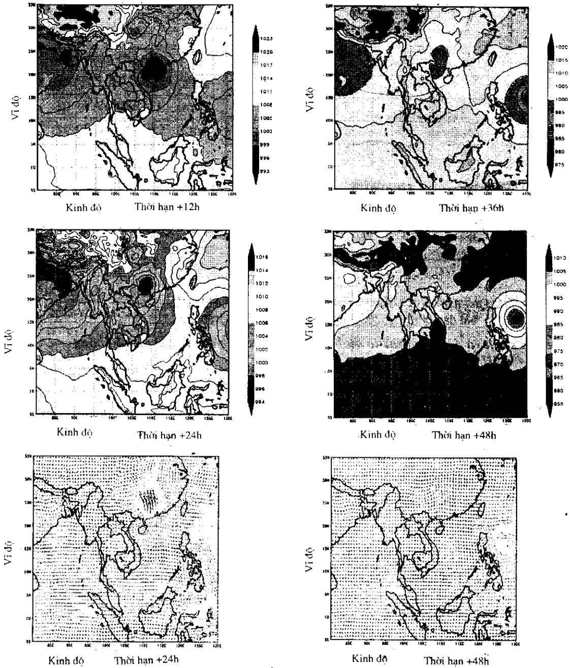
Hình 3.3. Bốn hình bên trên cùng biểu diễn trường áp mặt đất: +12h, +24h, +36h, +48h, hai hình dưới là trường gió trên mực 700mb: +24h và +48h, dự báo bằng HRM, bắt đầu 12Z 01 07 2001, bão DURIAN
