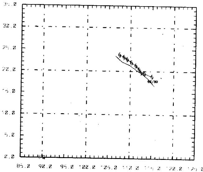
Hình 3.4. Quỹ đạo bão DURIAN dự báo +48h bằng VNUH/HRM, bắt đầu 00Z30062001, đồ hoạ bằng NCAR-Graphics
