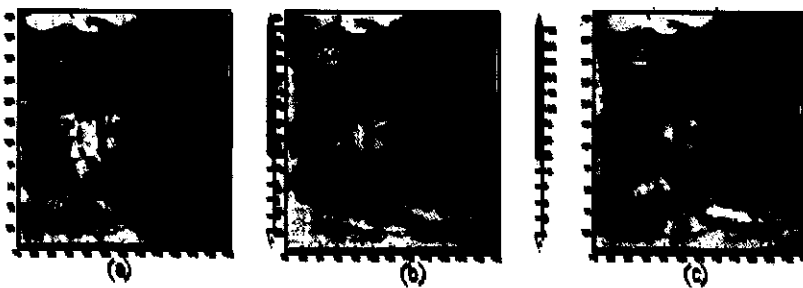
Hình 6. Trường lượng mưa (mm/tháng) trung bình các tháng mùa đông thời kỳ 1996-1998 mô phỏng bởi Reg+ERA40 (a), Reg+NNRP1 (b) và Reg+NNRP2 (c)
