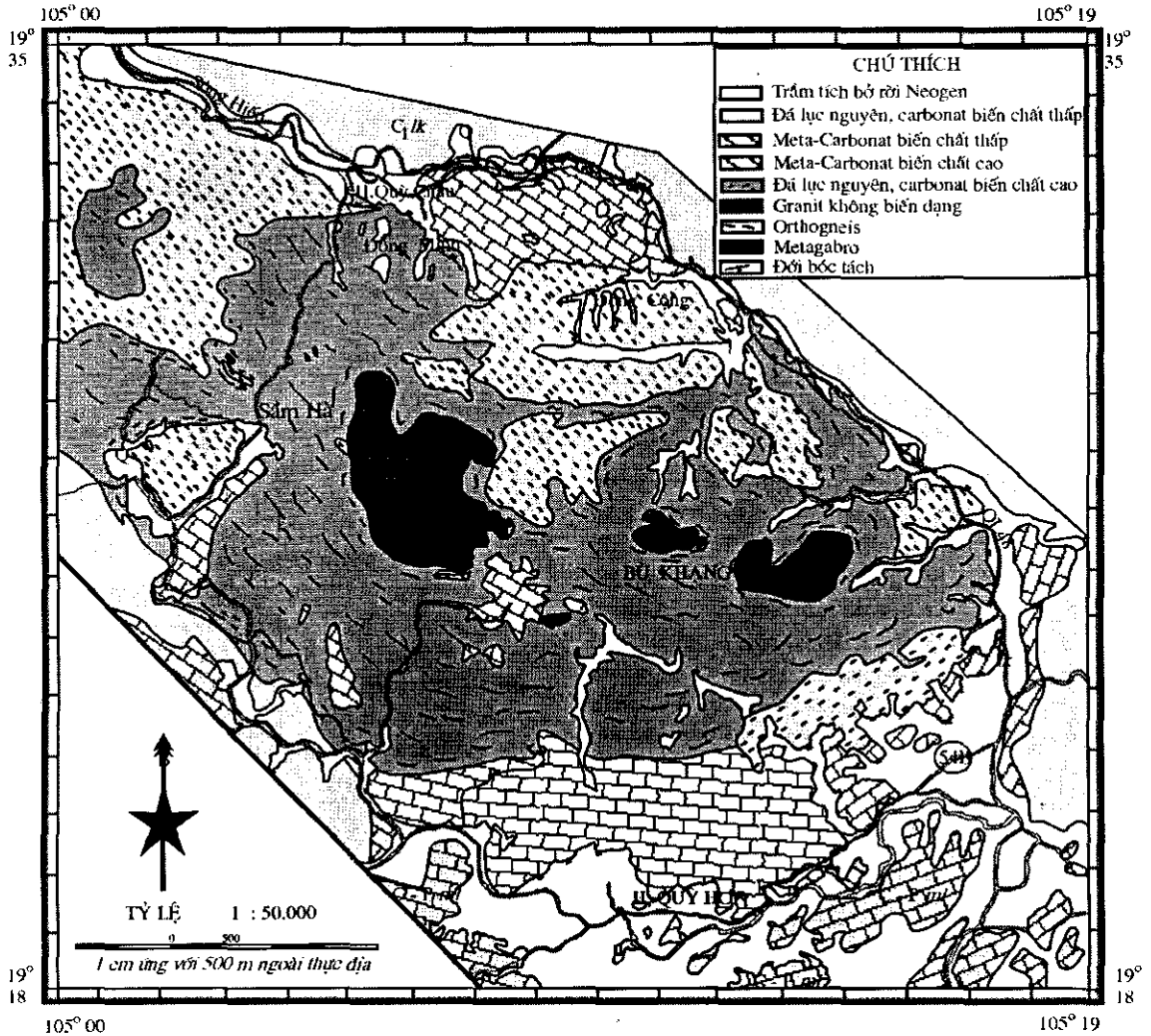
Hình 1. Sơ đồ địa chất khối Bù Khạng theo Lê Duy Bách (1998) và Jolivet et al (1999), được bổ sung tài liệu của các tác giả bài báo này
