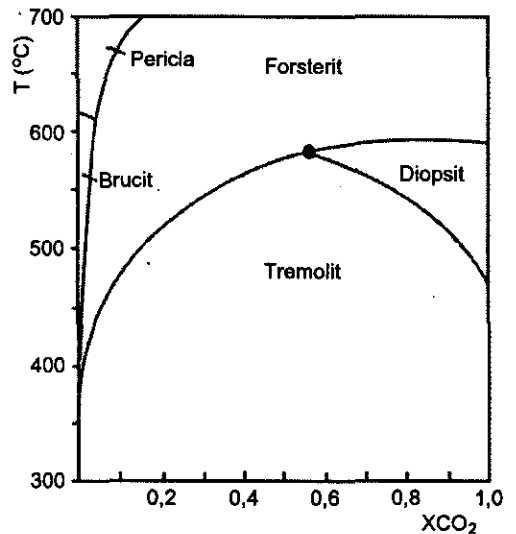
Hình 2. Biểu đồ xác định nhiệt độ T- X_{CO_2} và biểu đồ xác định áp suất P-T- X_{CO_2} cho đá hoa chứa tổ hợp cân bằng tremolit + diopsit + forsterit ở Quý Châu theo [M. Gottschalk và P. Metz (1984), ..Perkin (1986)]
