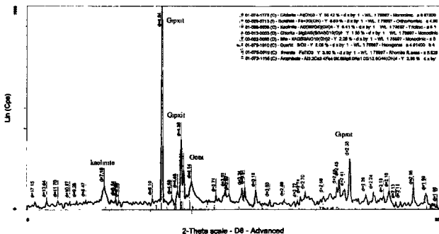
Hình 3. Biểu đồ phân tích XRD mẫu đất đỏ basalt Tân Rai - Lâm Đồng
