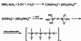
Hình 6. Phản ứng geopolimer hóa [11]
