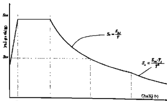
Hình 3. Phổ gia tốc theo ASCE 7
