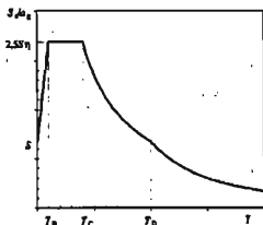
Hình 1. Dạng của phổ gia tốc
