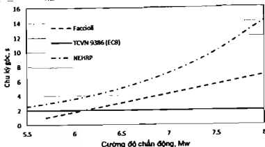
Hình 5. Biểu đồ quan hệ giữa chu kỳ góc của phổ chuyển vị và cường độ chấn động
