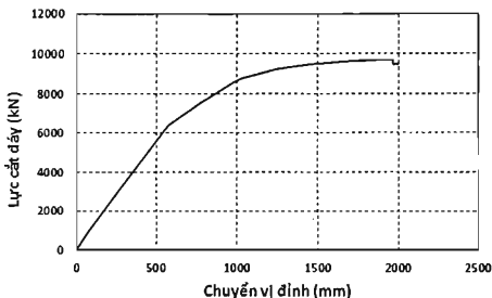
Hình 8. Đường cong khả năng của công trình
