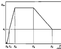
Hình 2. Phổ chuyển vị
