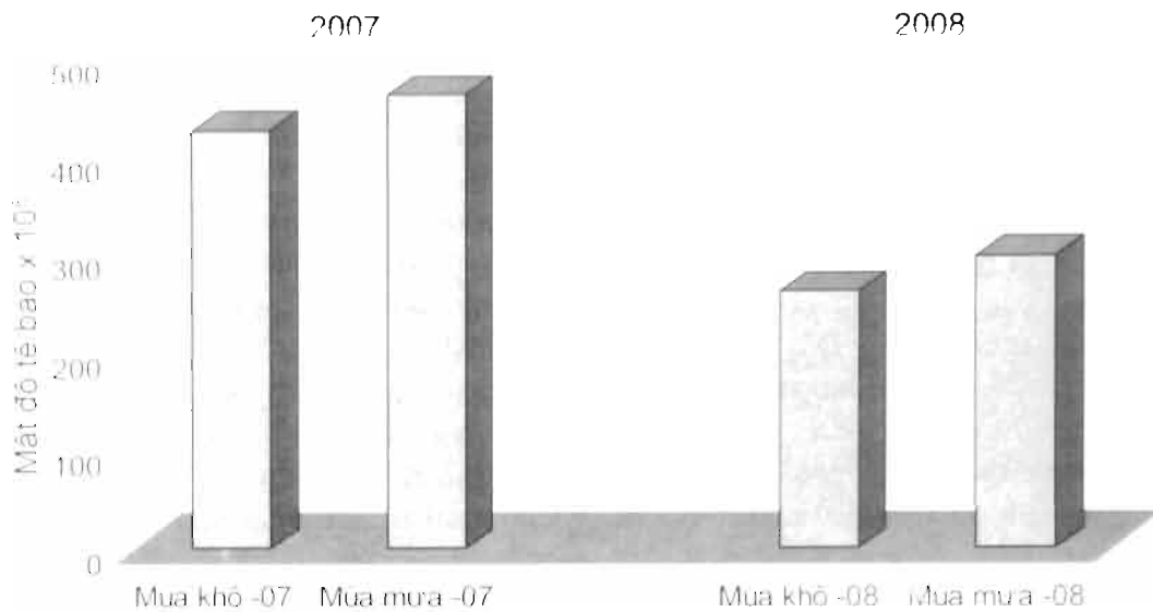
Hình 2. Biến động mật độ thực vật phù du trung bình trong hệ thống sông Nhuệ - Đáy theo mùa trong hai năm 2007 và 2008.
