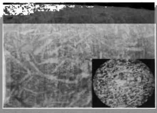
Ảnh 2. Đá vôi dolomit hóa có cấu trúc đẹp được tạo bởi các tinh thể calcit dạng que, kim, chùm, trên nền sọc dải đen xám sẫm. Ảnh lát mỏng phía dưới bên phải (ảnh của tác giả)
