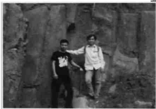
Ảnh 7. Các cột basalt có kích thước dao động 1,5-2m, thậm chí có cột cao 3-3,5m và đường kính 50-80cm lộ ra tại khu mỏ Làng Hạp, xã Đăk Tô Ma (ảnh của tác giả)
