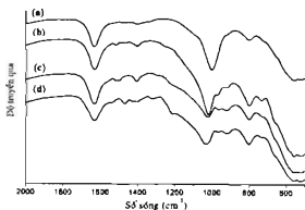
Hình 5. Phổ FT-IR của BDG trước (đường a) và sau khi hấp phụ chất màu Blue MERF (đường b), Yellow 3GF (đường c) và Red 3BF (đường d).
