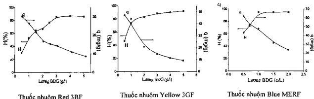
Hình 3. Ảnh hưởng của hàm lượng BDG tới khả năng hấp phụ các chất màu.
