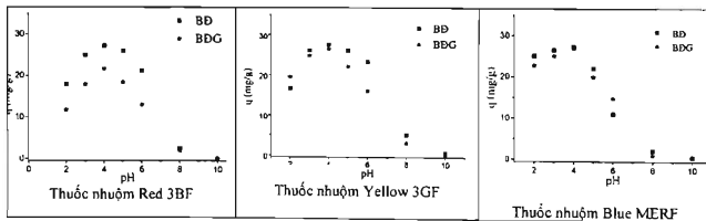
Hình 1. Ảnh hưởng của pH tới dung lượng hấp phụ chất màu của bùn đỏ.
