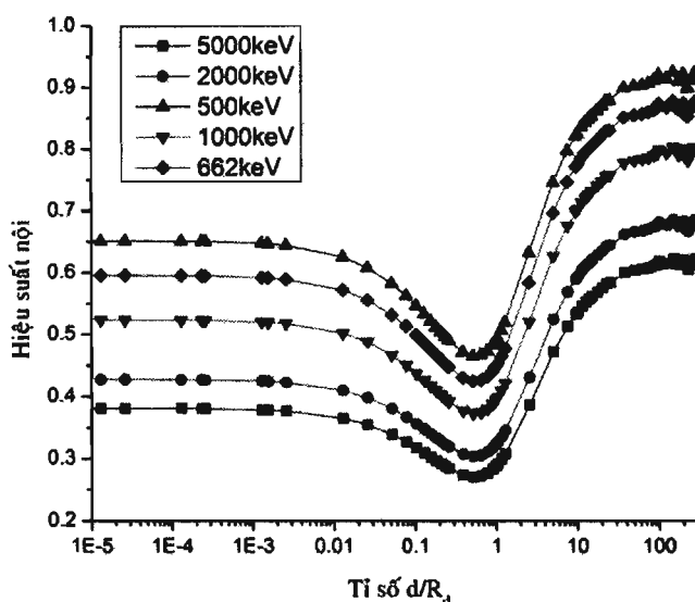
Hình 4. Sự phụ thuộc của hiệu suất nội theo tỉ số d/R_s
