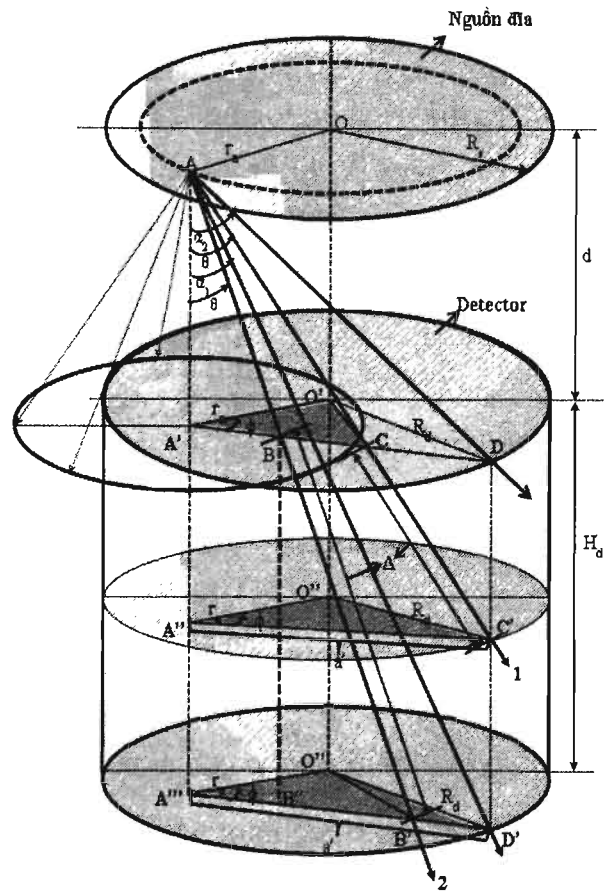
Hình 1. Nguồn đĩa đặt đồng trục với detector NaI(Tl)
